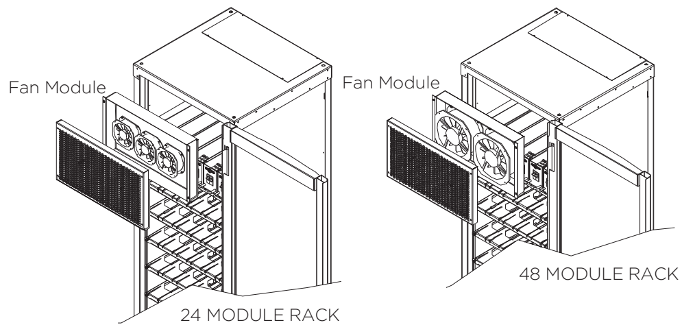
FIGURE 4. FAN MODULE
